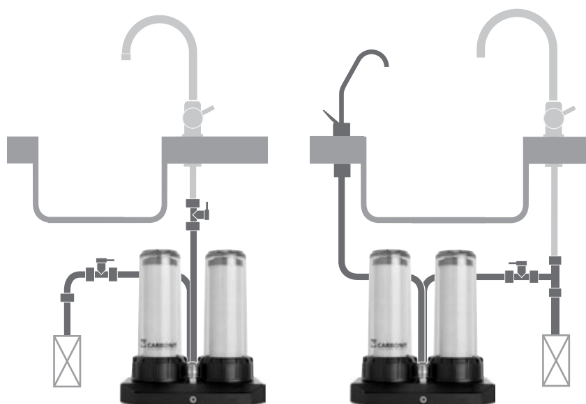
DUO Classique Schéma de montage
